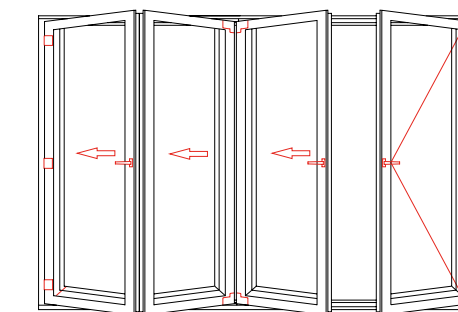
Puerta plegable
